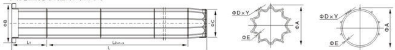
圆笼型滤袋框架外形图
