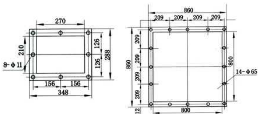
地脚尺寸
